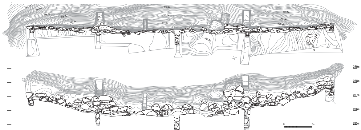
図 2-6 石垣 88 平面図・立面図
