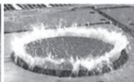
浮上防止ロック機能付きマンホール
