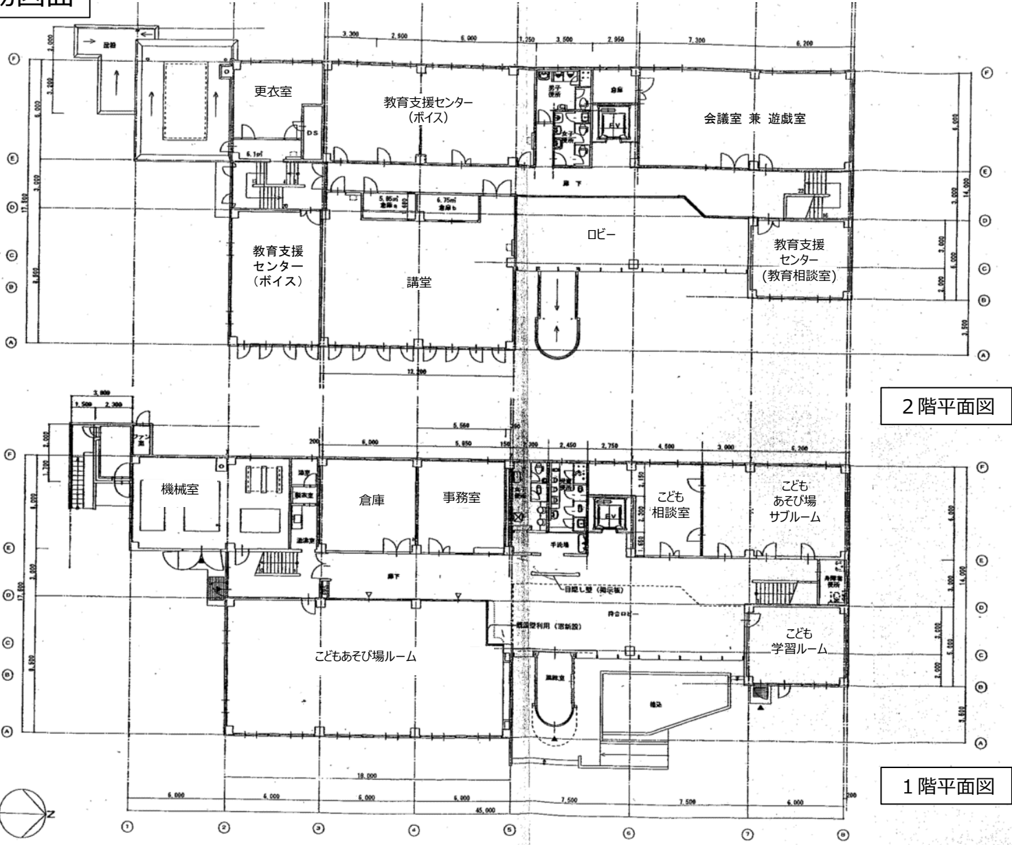
建物図面
