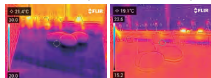
【床面のサーモカメラ写真（左：夏期、右：冬期）】
