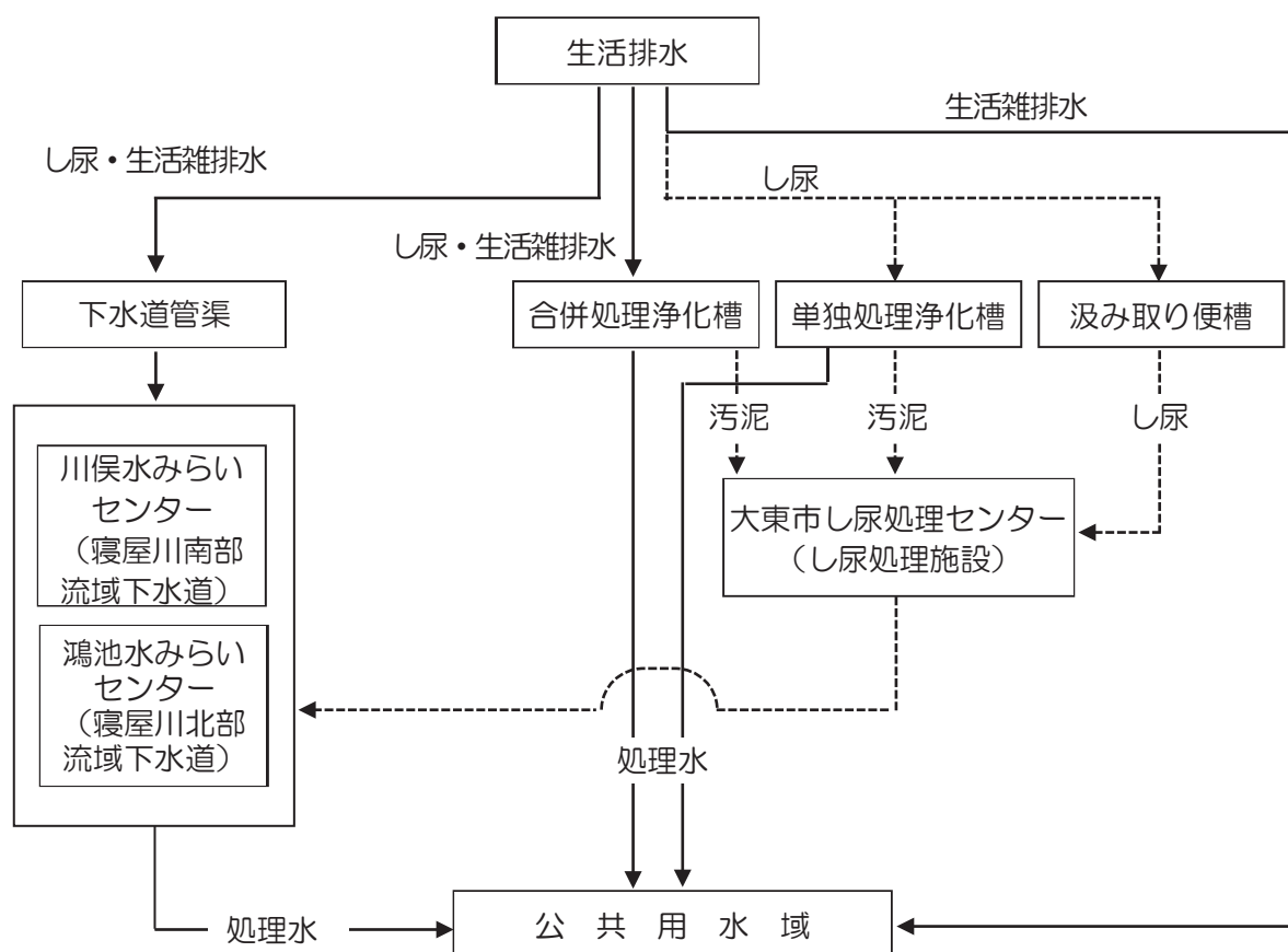
図 44 生活排水処理システムの現況
