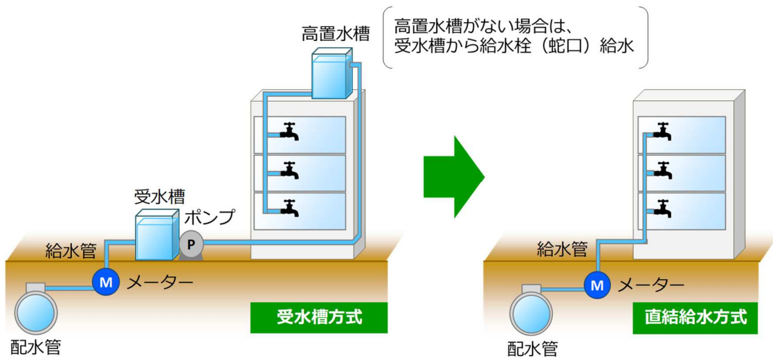
<受水槽方式と直結給水方式>
