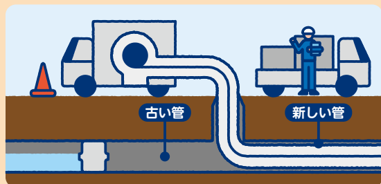
〈管更生工法による工事を行った管の中〉
